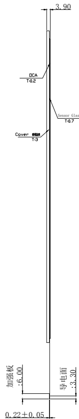
侧视图
