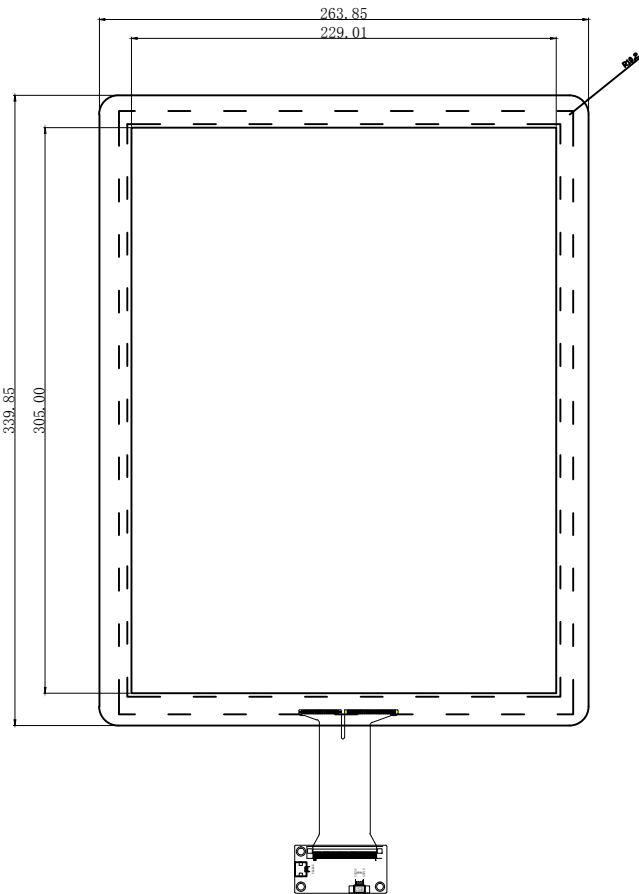
正视图
