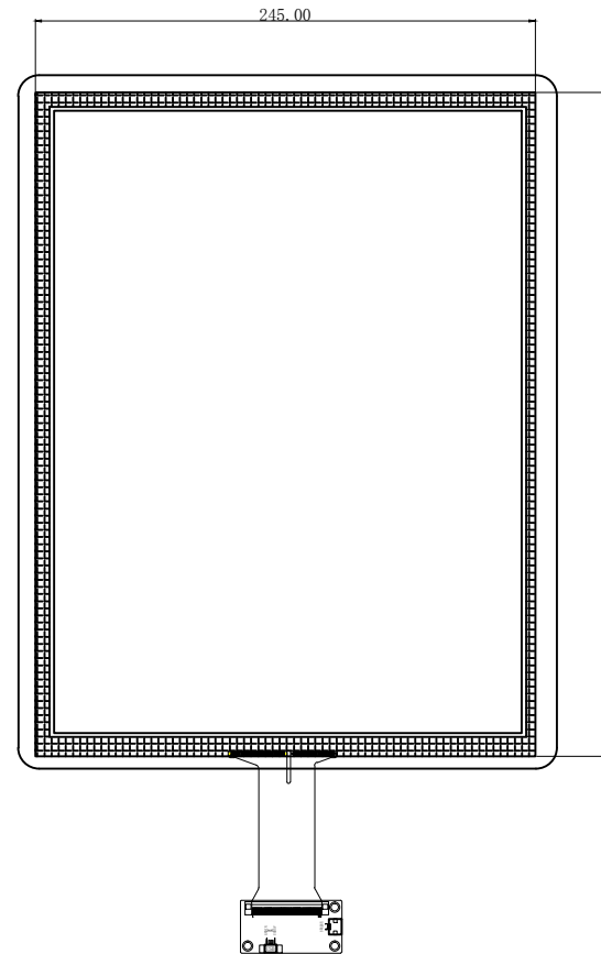
背视图
