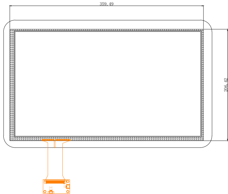
背视图
