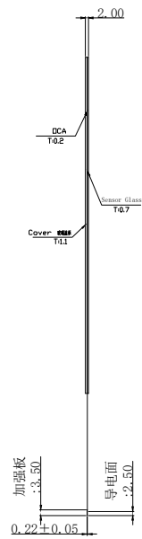
侧视图
