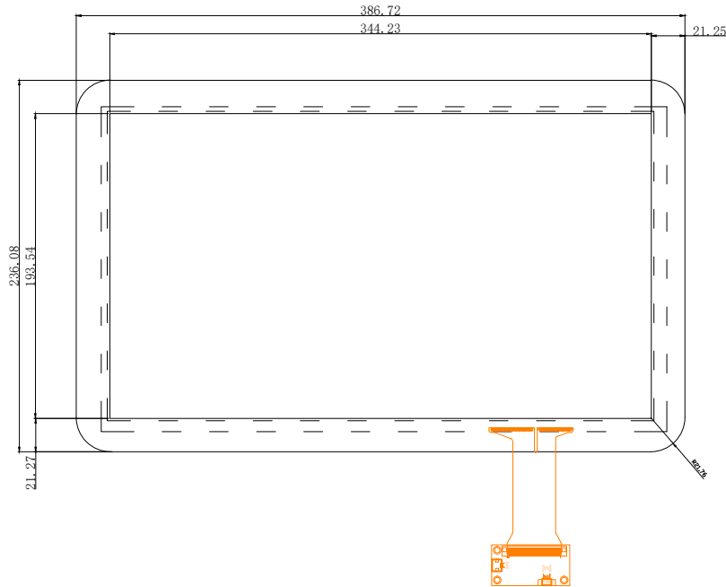
正视图
